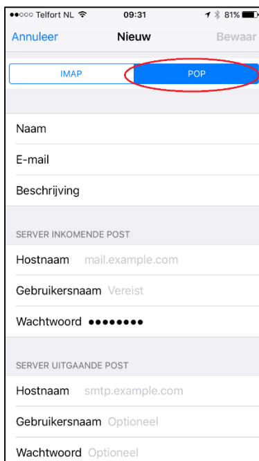
Afbeelding 5: Server
